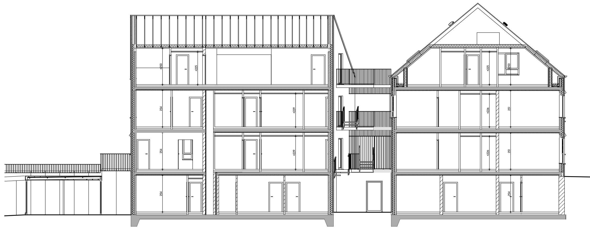
COUPE BB
