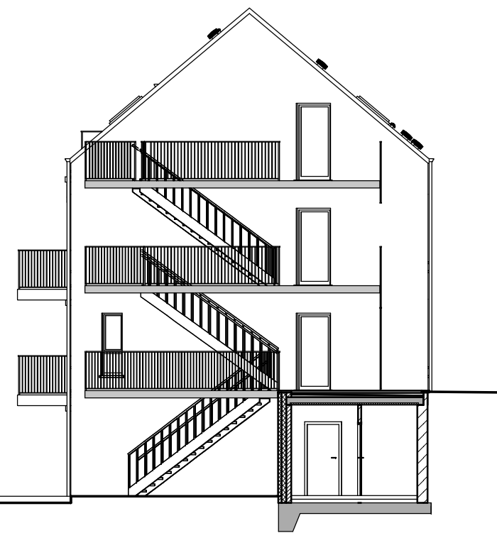
PIGNON DROIT BLOC 1
